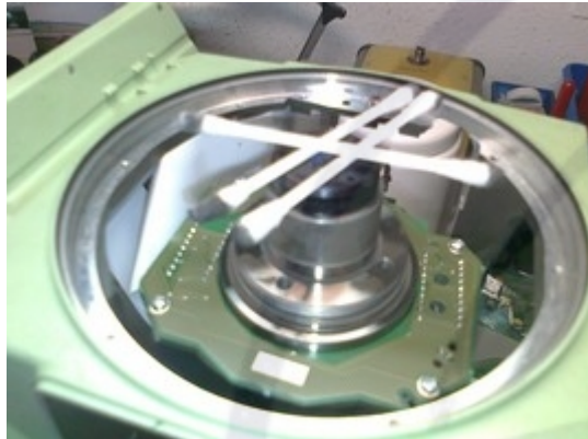
Alhidádé-alsórész megtisztítva
